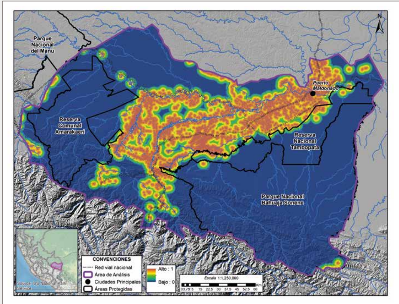
Figura 10. Tiempo de intervención
