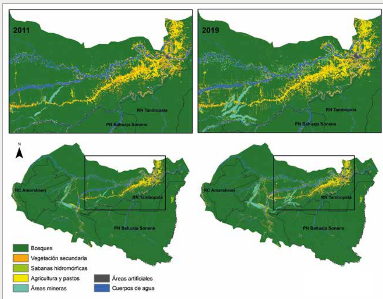
Figura 3. Variación espacial de los tipos de cobertura y usos del suelo entre 2011 y 2019 en el área de estudio; detalle de la sustitución de coberturas naturales por agricultura y pastos adyacentes a la vía Interoceánica, así como transformación de coberturas naturales a áreas mineras en el sector de La Pampa.
