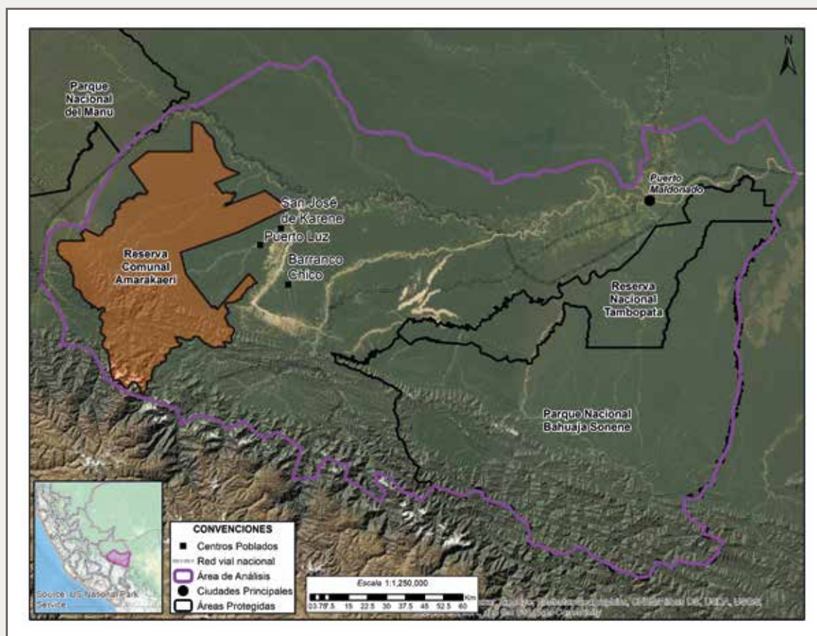
Figura 28. Localización de las comunidades de San José de Karene, Puerto Luz y Barranco Chico
