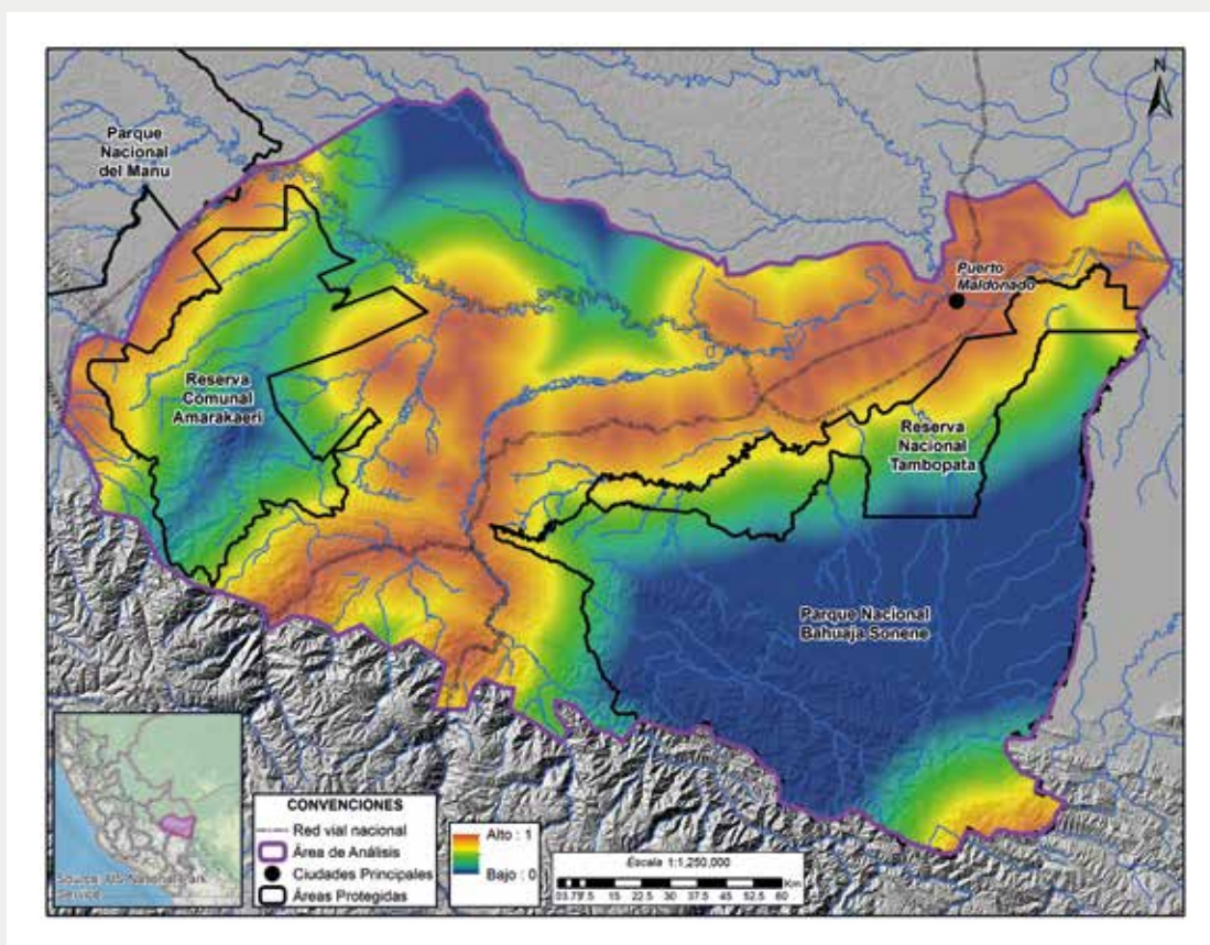
Figura 3. Distancia a centros poblados
