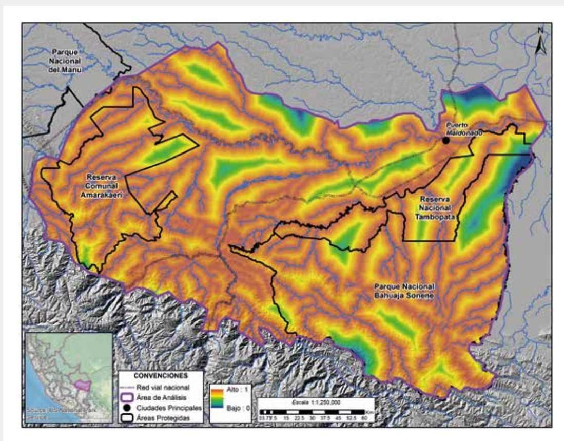
Figura 5. Distancia a ríos
