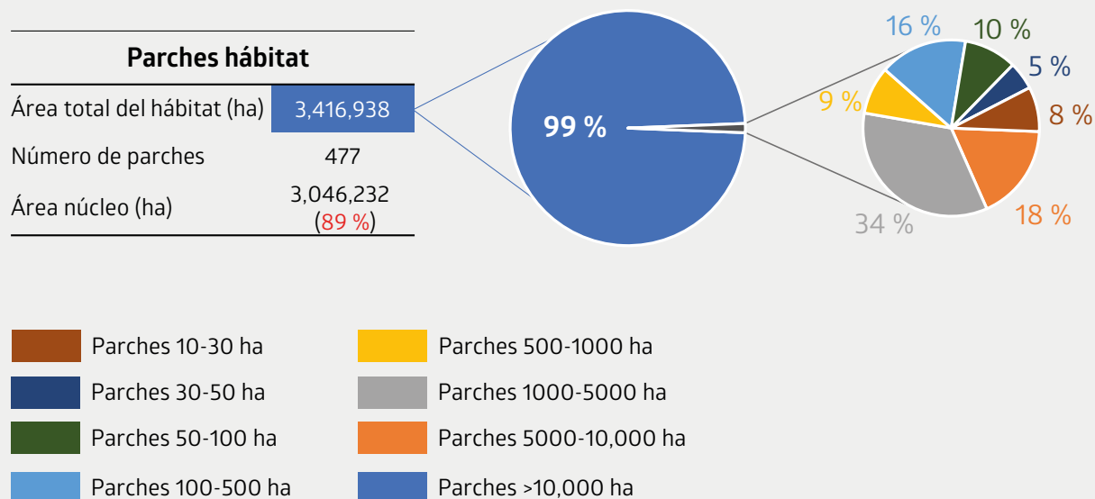
Figura 13. Nodos o parches hábitat para el grupo 1 de especies (majaz, batará grande y sajino)
