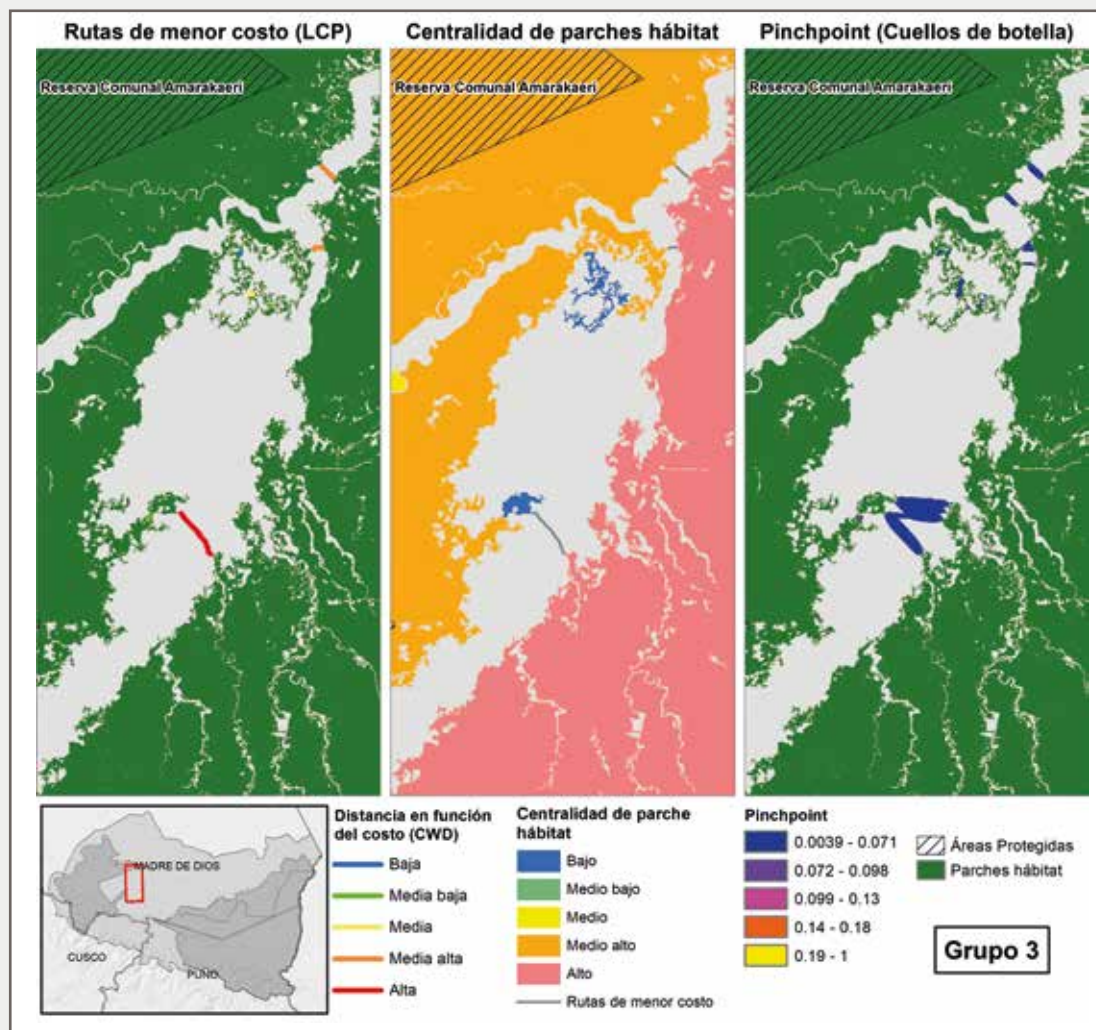
Figura 27. Rutas de menor costo de conectividad, centralidad de parches y “cuellos de botella” del grupo 3 ( Panthera onca , Puma concolor y Harpia harpyja ) para el sector de Delta 1, Puerto Luz, San José de Karene y Barranco Chico
