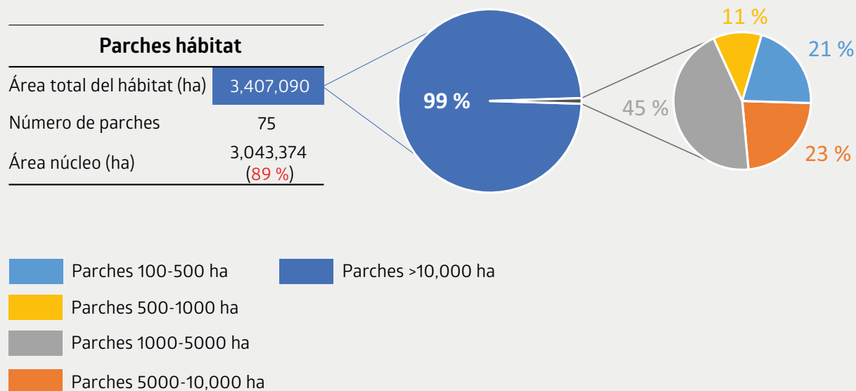
Figura 15. Nodos o parches hábitat para el grupo 3 de especies (jaguar, puma y águila harpía)
