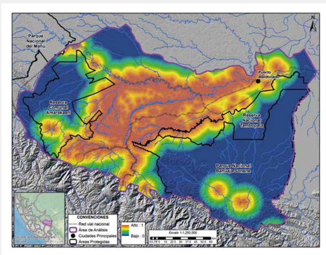
Figura 2. Distancia a minería, 2019
