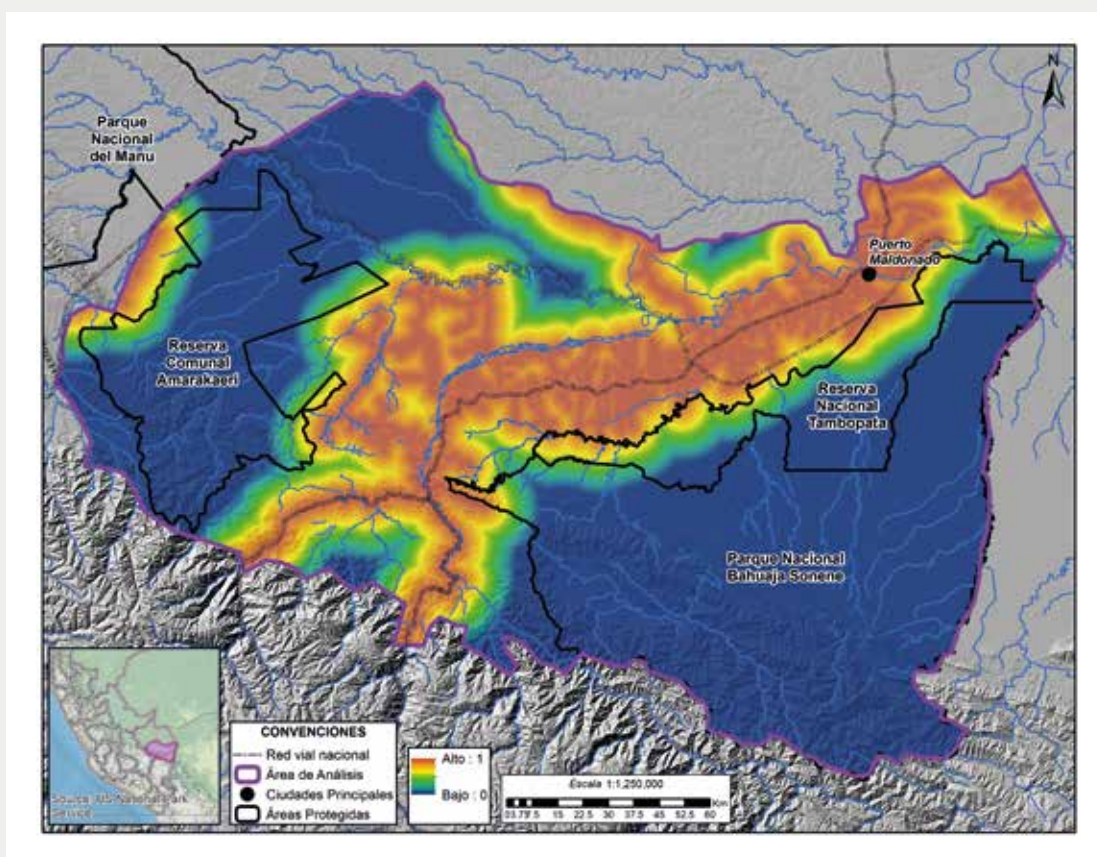
Figura 4. Distancia a vías
