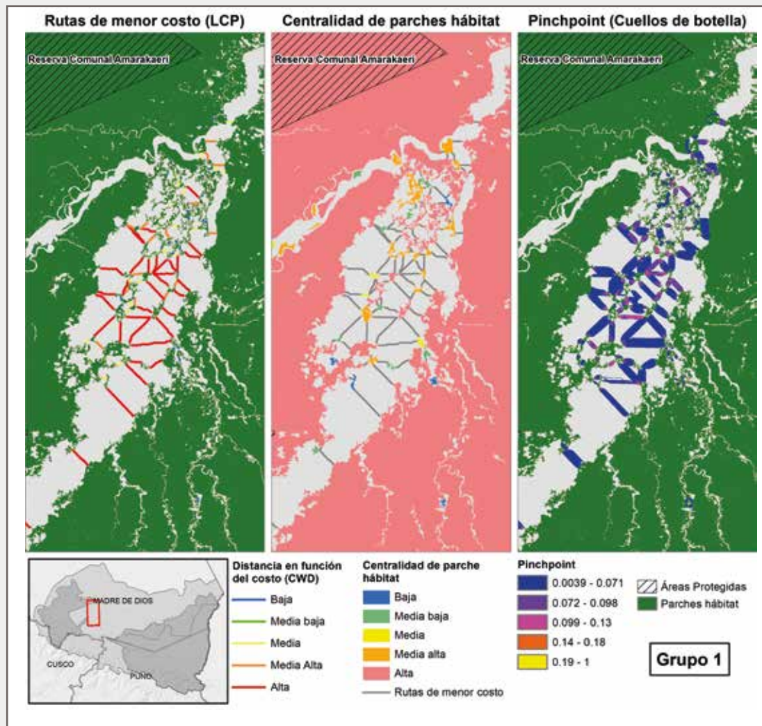
Figura 25. Rutas de menor costo de conectividad, centralidad de parches y “cuellos de botella” del grupo 1 ( Cuniculus paca , Taraba major y Dicotyles tajacu ) para el sector de Delta 1, Puerto Luz, San José de Karene y Barranco Chico
