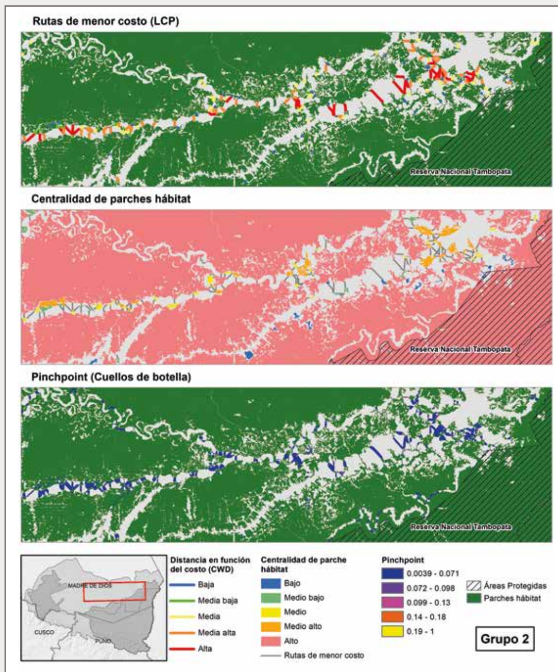
Figura 20. Rutas de menor costo de conectividad, centralidad de parches y "cuellos de botella" del grupo 2 ( Tapirus terrestris , Ateles chamek , Penelope jacquacu y Leontocebus weddelli ) para el sector de Puerto Maldonado y Vía Interoceánica
