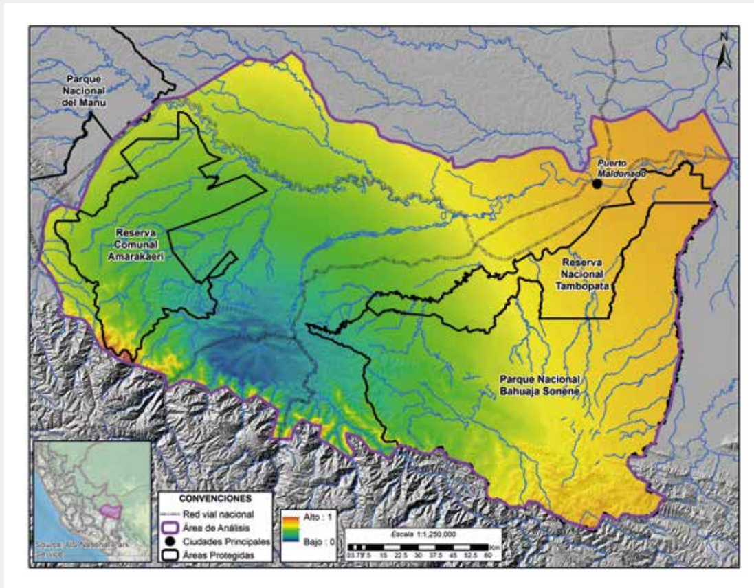
Figura 8. Índice de aridez
