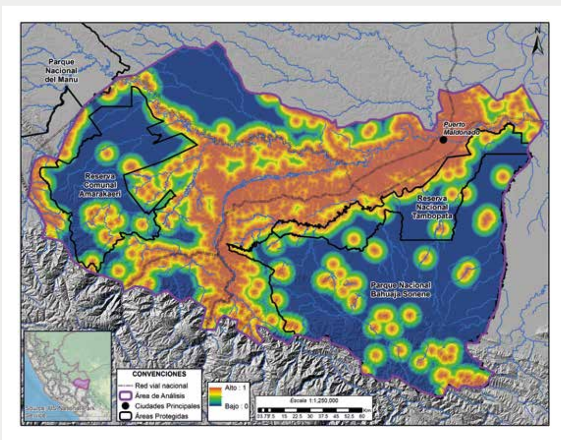
Figura 1. Distancia a pastos y agricultura, 2019
