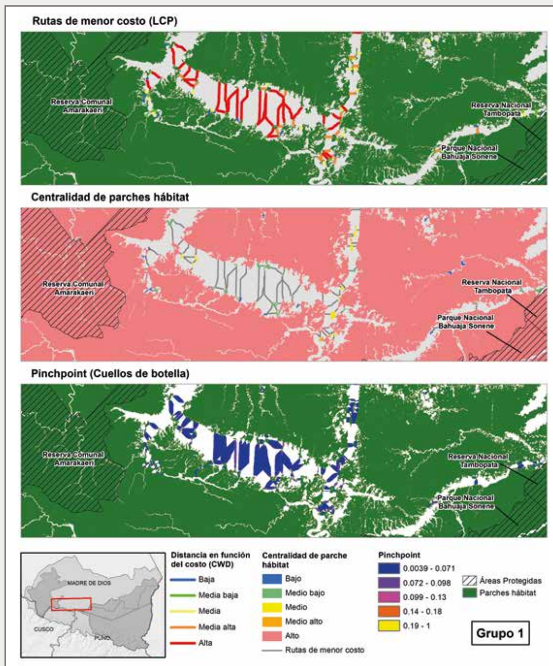
Figura 22. Rutas de menor costo de conectividad, centralidad de parches y "cuellos de botella" del grupo 1 ( Cuniculus paca , Taraba major y Dicotyles tajacu ) para el sector de Huepetuhe y Mazuko
