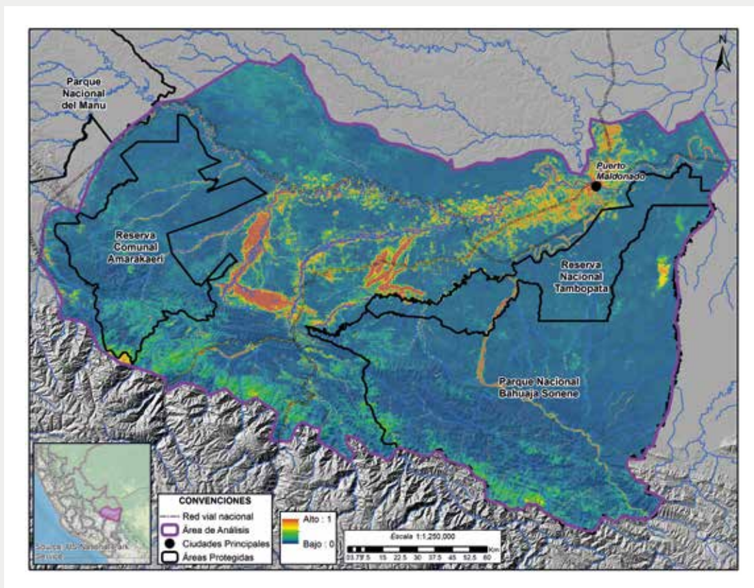
Figura 7. Índice de biomasa
