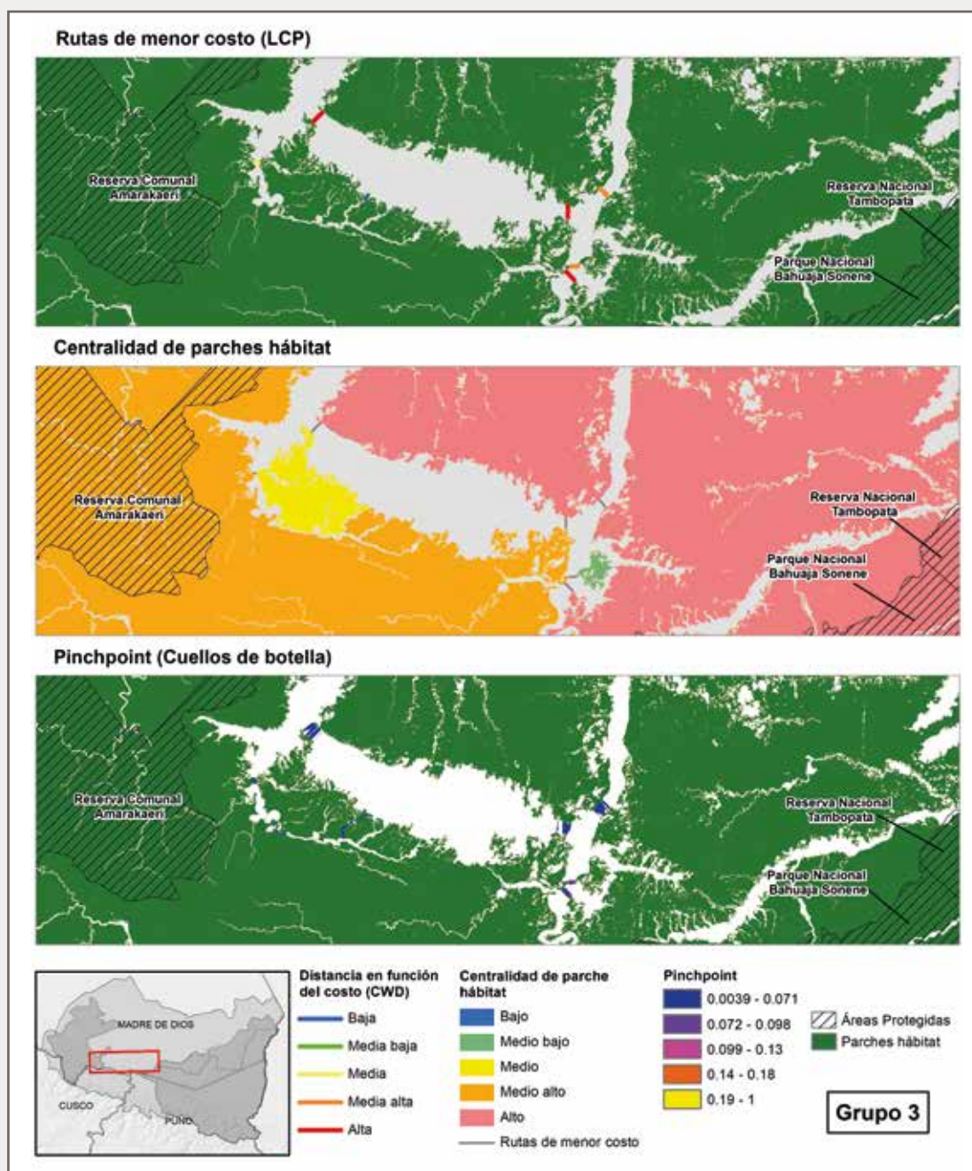
Figura 23. Rutas de menor costo de conectividad, centralidad de parches y "cuellos de botella" del grupo 2 ( Tapirus terrestris , Ateles chamek , Penelope jacquacu y Leontocebus weddelli ) para el sector de Huepetuhe y Mazuko
