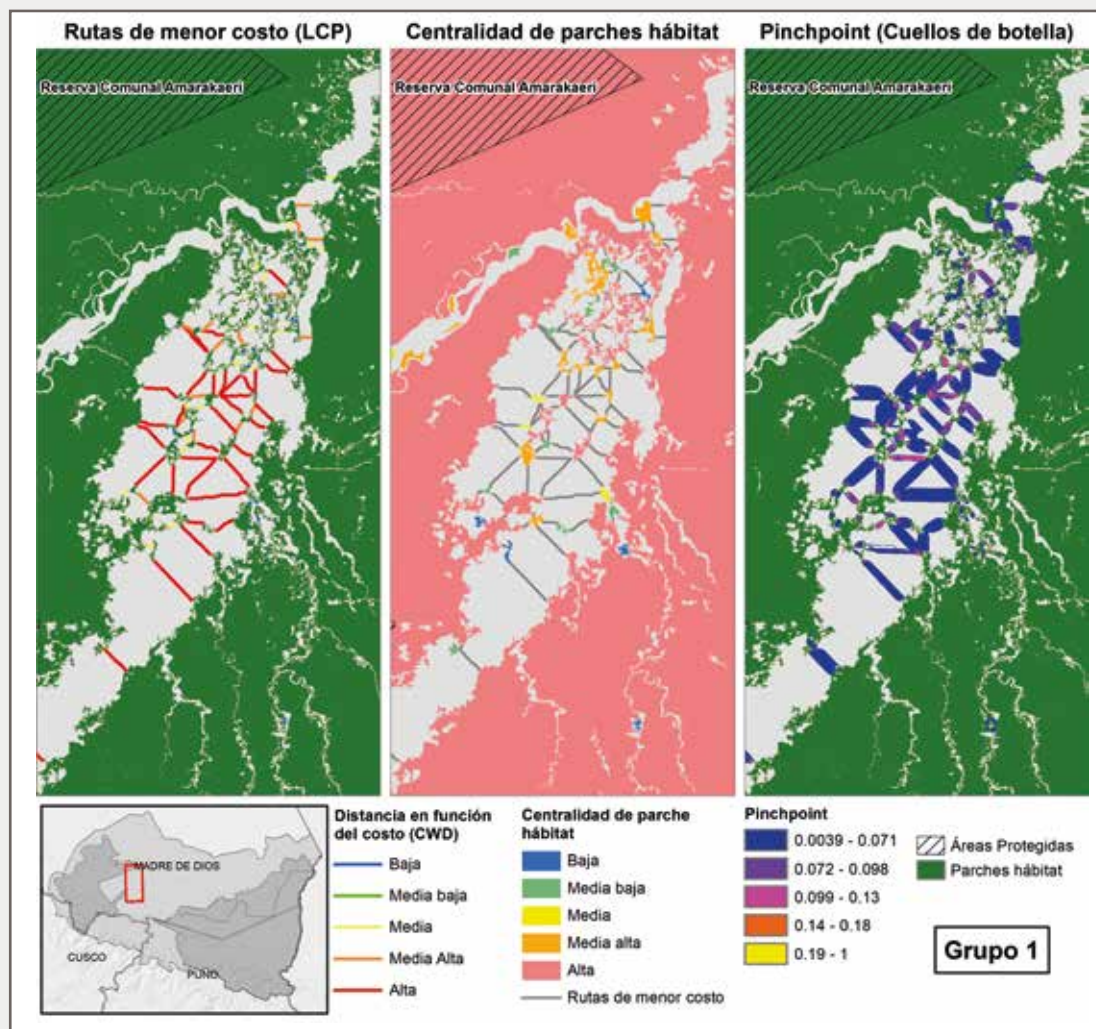
Figura 26. Rutas de menor costo de conectividad, centralidad de parches y “cuellos de botella” del grupo 2 ( Tapirus terrestris , Ateles chamek , Penelope jacquacu y Leontocebus weddelli ) para el sector de Delta 1, Puerto Luz, San José de Karene y Barranco Chico
