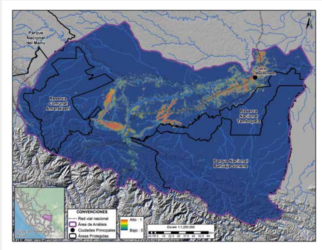
Figura 6. Índice de fragmentación
