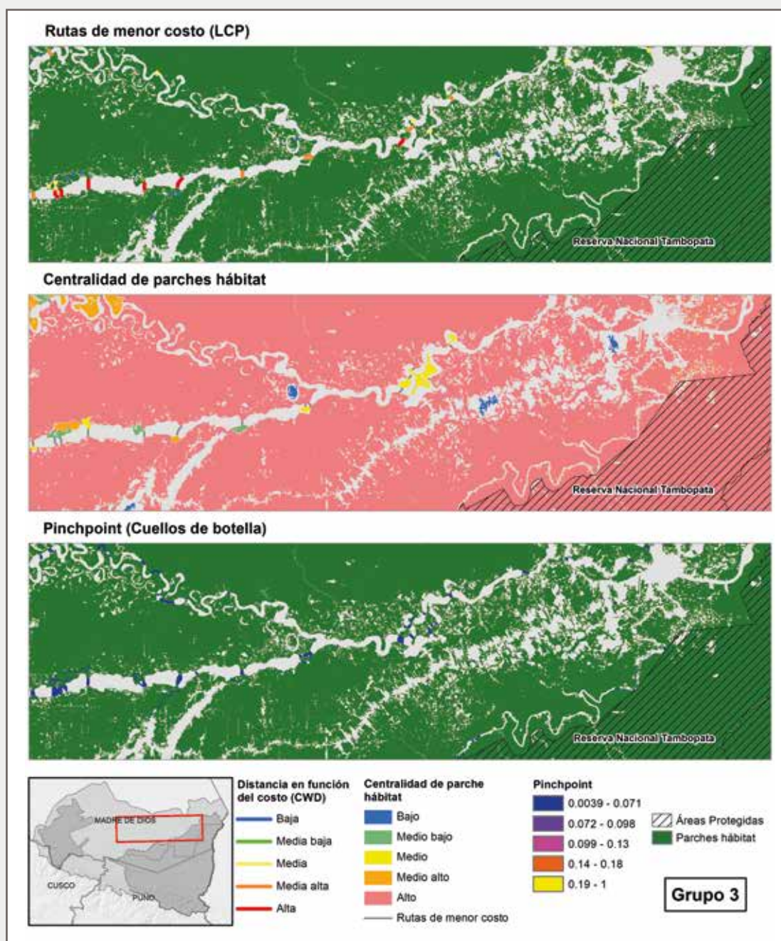
Figura 21. Rutas de menor costo de conectividad, centralidad de parches y "cuellos de botella" del grupo 3 ( Panthera onca , Puma concolor y Harpia harpyja ) para el sector de Puerto Maldonado y Vía Interoceánica
