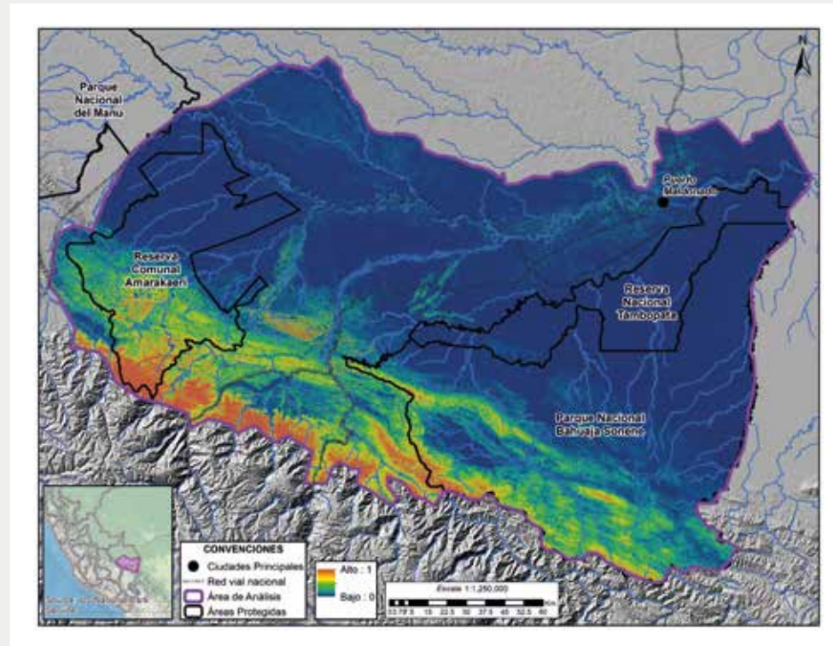
Figura 10. Ecuación de pérdida de suelo universal revisada
