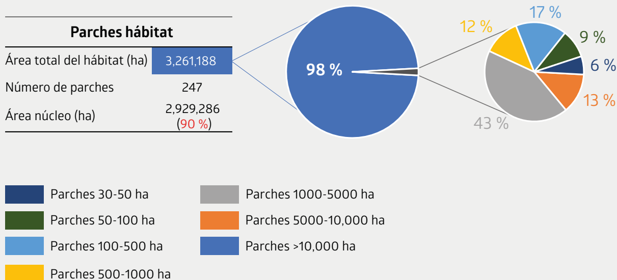
Figura 14. Nodos o parches hábitat para el grupo 2 de especies (tapir, maquisapa, pucacunga y pichico)
