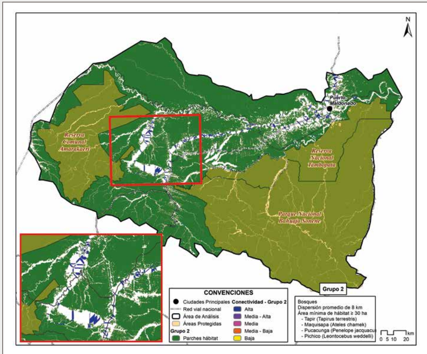
Figura 17. Corredores de conectividad funcional para el grupo 2 ( Tapirus terrestris , Ateles chamek , Penelope jacquacu y Leontocebus weddelli )
