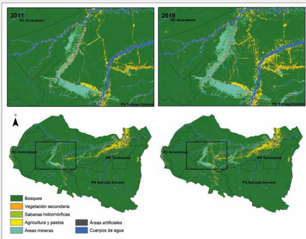
Figura 2. Variación espacial de los tipos de cobertura y usos del suelo entre 2011 y 2019 en el área de estudio; detalle de la sustitución de coberturas naturales por agricultura y pastos; así como transformación de coberturas naturales a áreas mineras entre los ríos Madre de Dios, Punkiri e Inambari.
