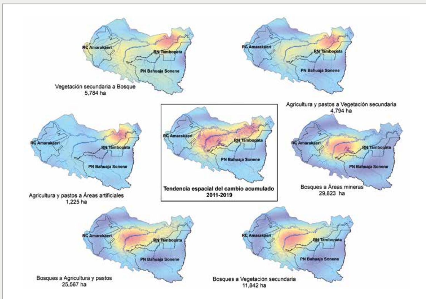
Figura 4. Tendencia espacial del cambio entre 2011 y 2019 de los procesos de mayor magnitud en el área de estudio (se muestran en color rojo las zonas con mayor tendencia de cambio entre coberturas y usos del suelo, y en color azul, las zonas con menor tendencia de cambio)
