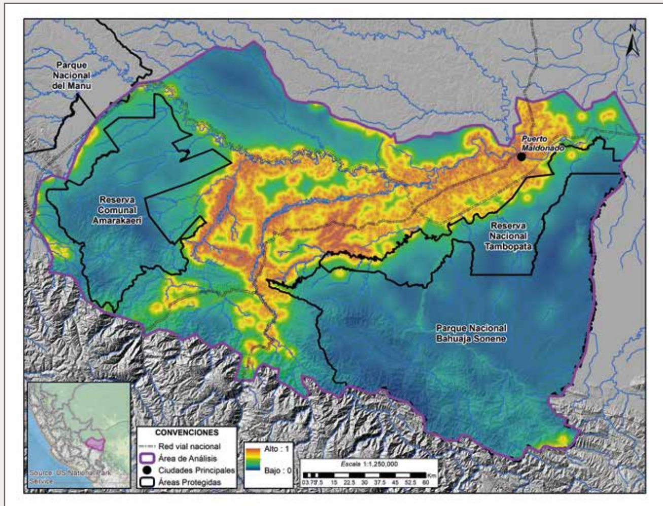
Figura 12. Índice espacial de huella humana
