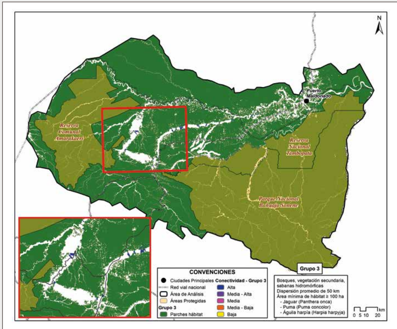
Figura 18. Corredores de conectividad funcional para el grupo 3 ( Panthera onca , Puma concolor y Harpia harpyja )
